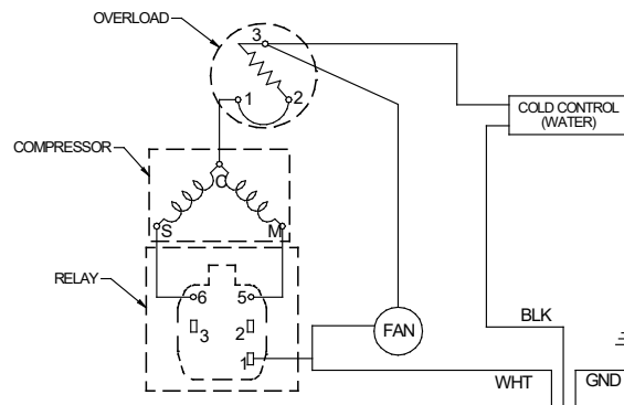
Fig. 14 115V Wiring Diagram
