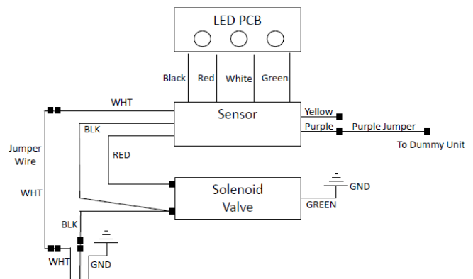
WIRING DIAGRAM - EZO 220V
